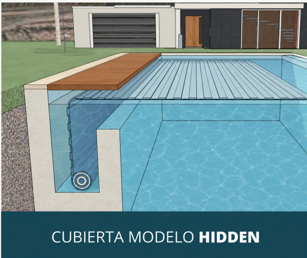
El conjunto de recogida se aloja bajo una tapa integrada al extremo de la piscina.
