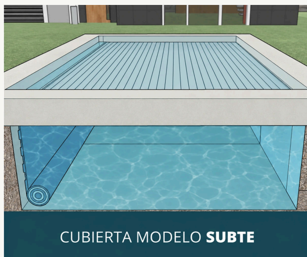
Las láminas se recogen en un eje sumergido, fijado a las paredes laterales.
